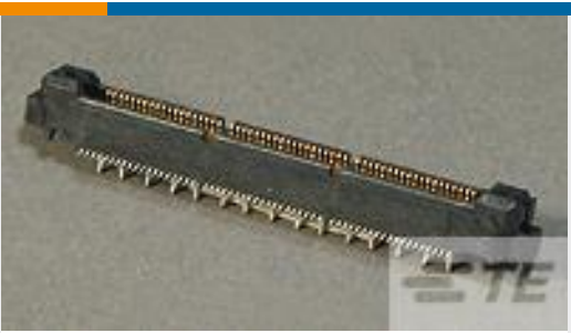
TE 产品编号 767116-3 MICT,260PLG,114,ASY,.025,AUPLT
