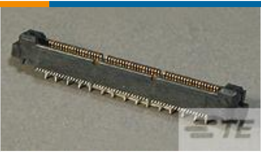
TE 产品编号 767117-3 MICT,260,PLG,114,ASY,.025,PDNI
