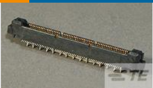
TE 产品编号 1-767118-0 MICT,PLG,114,ASY,.025,TAPE PKG
