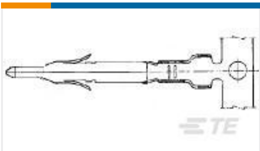
TE 产品编号170363-3 MINI UNIVERSAL M-N-L PIN LP
