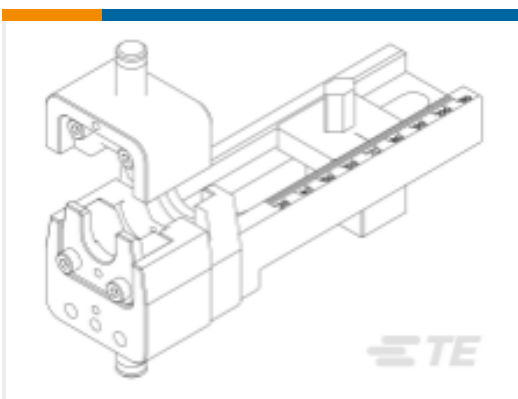
TE 产品编号2234154-1 DIE SET2 IPT-180-1/2/3P F 35MM2
