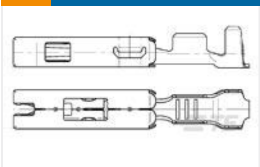
TE 产品编号929025-2 1.5MM SFC
