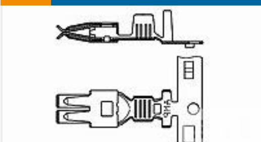
TE 产品编号963894-1 STECKHUELSE 6,3
