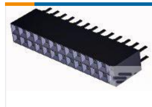
TE 产品编号1-534998-3 26 MODIV VRT DR CE 100/125
