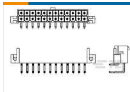
TE 产品编号1586044-6 6P VAL-U-LOK R/A HDR SCR MT V0
