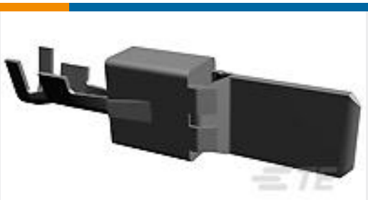
TE 产品编号963766-2 TAB 9.5x1.2 CONTACT CF SRC Sn
