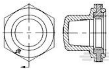
TE 产品编号174414-000 SO63-2-55-20-90
