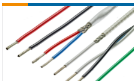
TE 产品编号3318953001 44A1161-22-0/1/2/3/4/5-9
