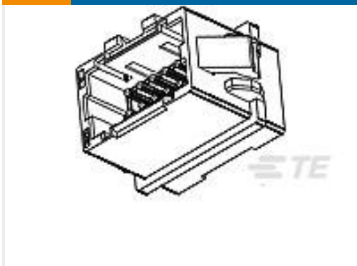
TE 产品编号2-292216-8 MINI CT D/R RELAY 28P V NAT
