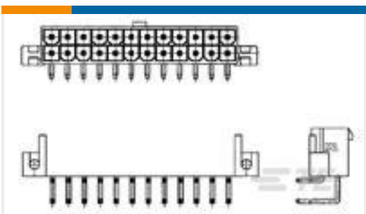
TE 产品编号2-1586043-2 22P VAL-U-LOK R/A HDR SCRMT V2
