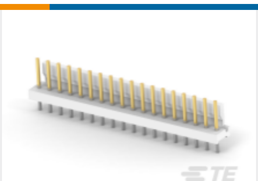
TE 产品编号 4-644760-8 18P MTA156 HDR ASSY FL ST LF
