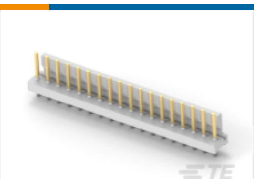
TE 产品编号 4-641209-8 18P MTA156 HDR ASSY FL ST LF
