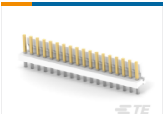
TE 产品编号 4-644759-8 18P MTA156 HDR ASSY STR LF
