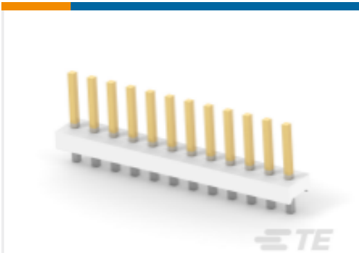
TE 产品编号 4-641203-2 12P MTA156 HDR ASSY PL 30AU LF
