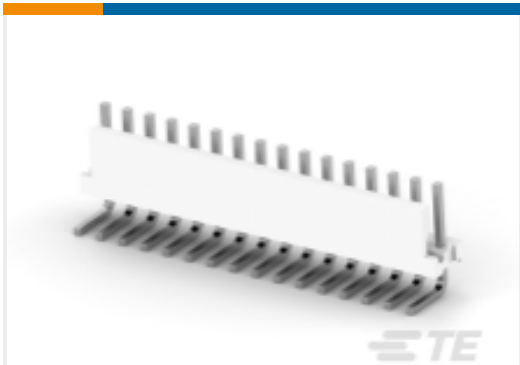
TE 产品编号 4-644755-6 16P MTA156 HDR ASSY SQ RARB F/L
