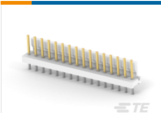
TE 产品编号 4-644760-6 16P MTA156 HDR ASSY FL ST LF
