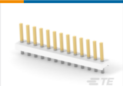
TE 产品编号 4-641203-3 13P MTA156 HDR ASSY PL 30AU LF
