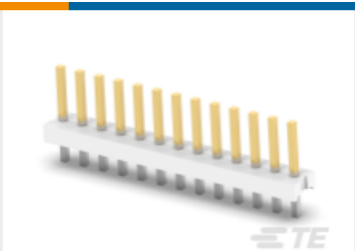
TE 产品编号 4-644756-3 13P MTA156 HDR ASSY STR AU LF
