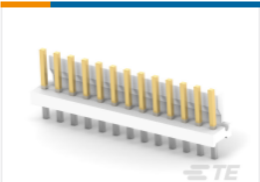
TE 产品编号 4-644759-3 13P MTA156 HDR ASSY STR LF
