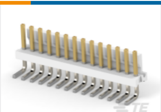
TE 产品编号 4-644768-4 14P MTA156 HDR ASSY F/L SQ LF
