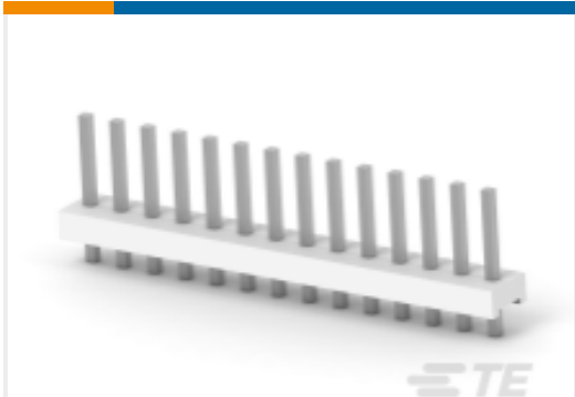
TE 产品编号 4-641113-4 14P MTA156 HDR ASSY 15AU LF
