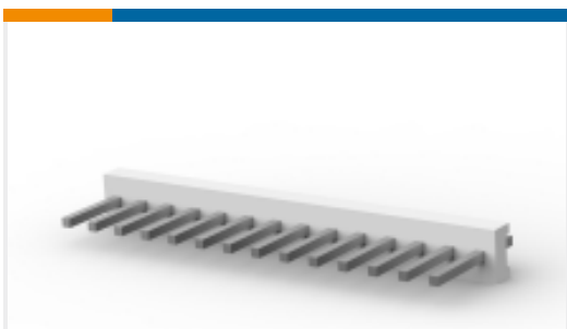
TE 产品编号 1-640383-4 14P MTA156 HDR ASSY STR SQ SN
