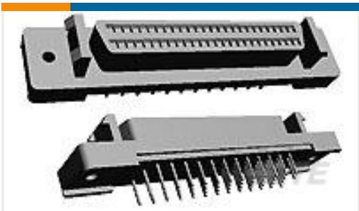
TE 产品编号749721-3 28 50SR VERT RCPT ASSY
