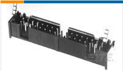
TE 产品编号1-1761606-6 IDC LOW PRO HDR 60P VERT LG LA
