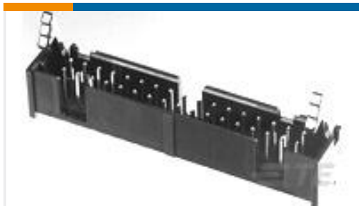
TE 产品编号1-1761606-5 IDC LOW PRO HDR 50P VERT LG LA
