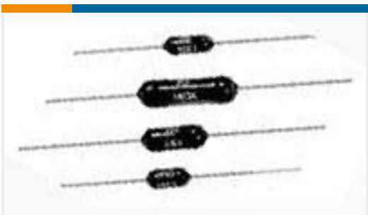
TE 产品编号3-1879675-2 H8 26K1 0.1% 25PPM
