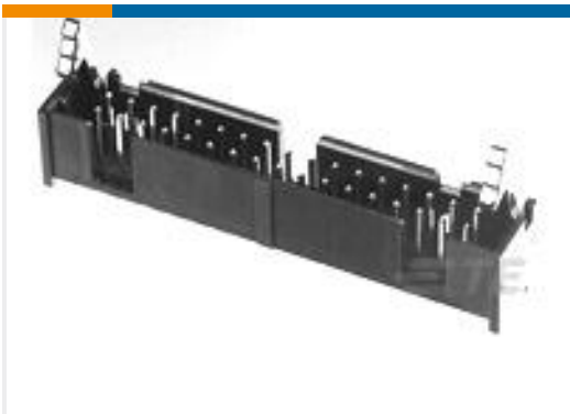
TE 产品编号2-1761606-6 IDC LOW PRO HDR 16P VERT LG LAT BLUE
