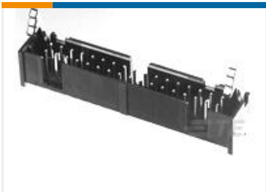
TE 产品编号2-1761606-3 IDC LOW PRO HDR 10P VERT LG LAT BLUE
