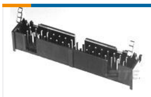
TE 产品编号1761608-3 IDC LOW PRO HDR 10P VERT SHT L
