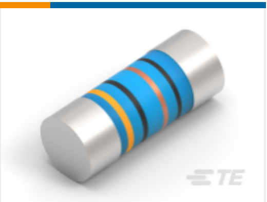
TE 产品编号6-2176314-1 MELF SMA_A 15K 1% 50PPM 0102 0.3 W
