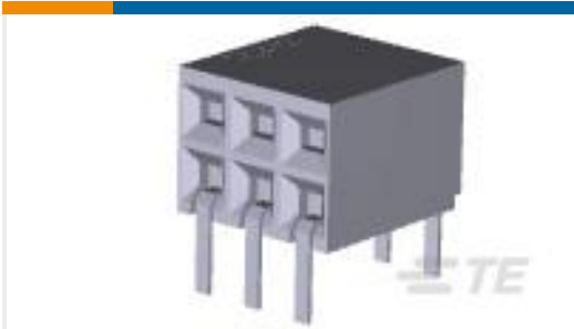
TE 产品编号 6-535512-2 06 MODII HORZ DR CE EESS .100
