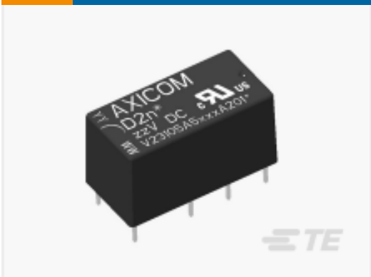
TE 产品编号1393793-2 V23105A5306A201
