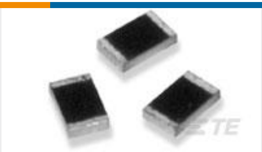
TE 产品编号1-1625868-6 RP 2A 0.25W 5K62 0.1% 25PPM 1K RL
