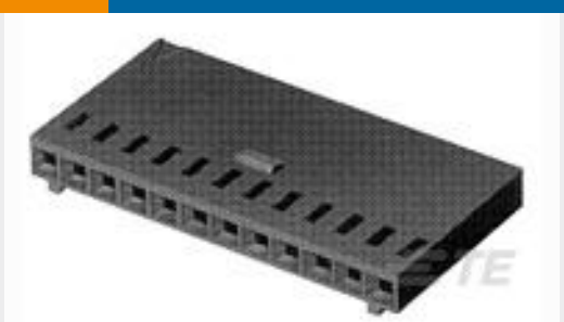
TE 产品编号102241-6 08 MODIV HSG COMP SR .100 POL
