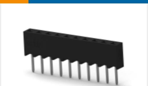
TE 产品编号1-2314868-0 10P,2MM,BB,REC,SRVT,2.0,0.1AU,TB, W/CP
