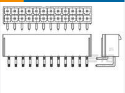
TE 产品编号1586863-4 4P VAL-U-LOK R/A HDR GW
