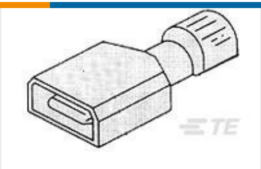
TE 产品编号3-520106-2 ULTRA-FAST 250 ASY TAB 16-14 AWG TPBR
