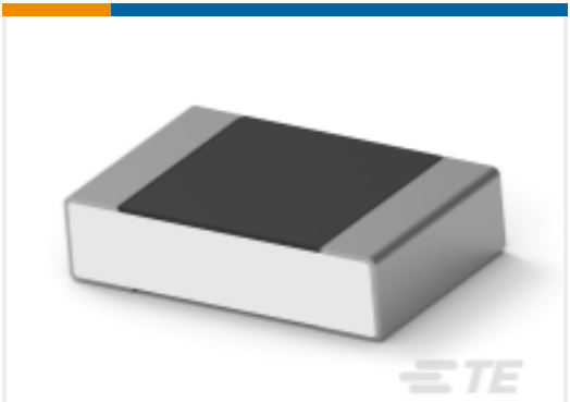
TE 产品编号2-2176376-4 RQ 0805 21K5 0.1% 10PPM 1K RL
