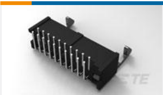
TE 产品编号1-1761607-1 IDC LOW PRO HDR 34P RA LG LAT
