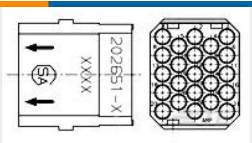
TE 产品编号202651-4 SKT MODULE, 23 POSN, G-SERIES
