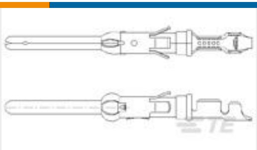
TE 产品编号163089-9 PIN TYPE III CONTACT SIZE 16
