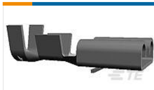
TE 产品编号160913-1 FF 250 REC 2.5-4.0MM2 BR
