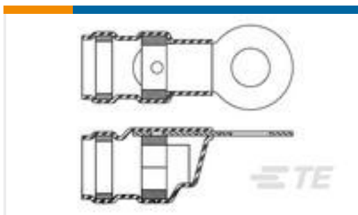
TE 产品编号696908-000 W-062-09
