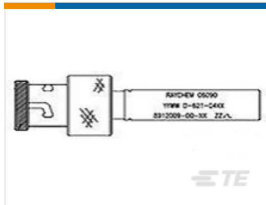
TE 产品编号106556-000 D-621-0653
