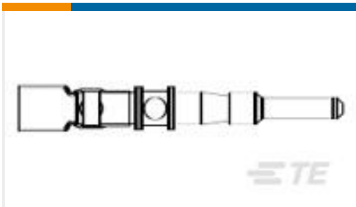
TE 产品编号601019-000 D-602-17
