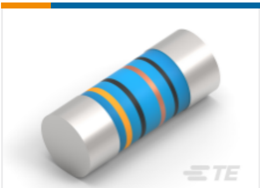
TE 产品编号1-2176315-5 MELF SMA_A 1K5 0.1% 15PPM 0204 0.4W
