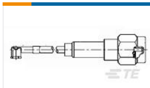
TE 产品编号1064391-1 9950 4200 01
