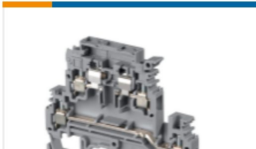
TE 产品编号 1SNA115604R2100 M4/8.D2.SF
