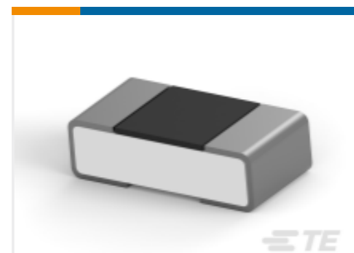
TE 产品编号5-2176359-3 RQ 0402 140R 0.1% 10PPM 1K RL
