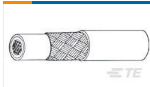
TE 产品编号3874483002 44A1111-24-2L-9
