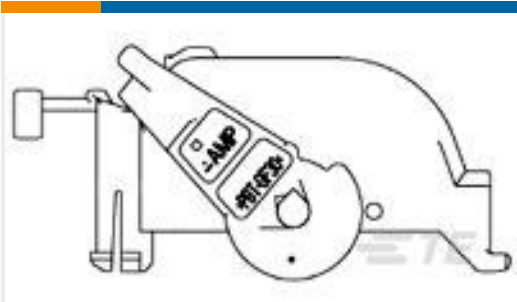
TE 产品编号 1473255-1 MQS 40P LEVER(L) ASSY
