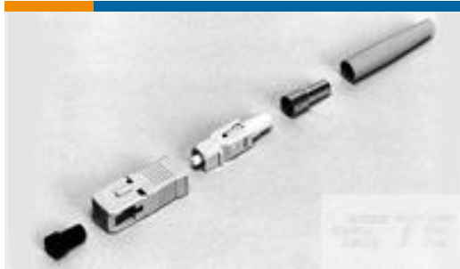
TE 产品编号 5504930-1 KIT,CONN,MM,SC 128UM 2.4MM SP
