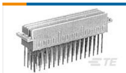
TE 产品编号167771-1 64P.IEC-G FEM.CONN.
