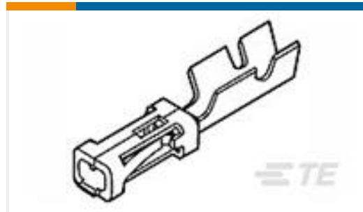
TE 产品编号167023-2 MOD-4 REC.CONTACT
