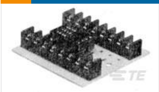
TE 产品编号1393837-1 27E460=SOCKET,R10,,ASSY,2 POLE
