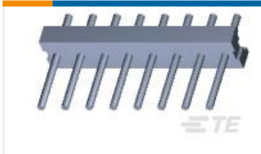
TE 产品编号3-641203-8 08P MTA156 HDR ASSY PL 30AU LF
