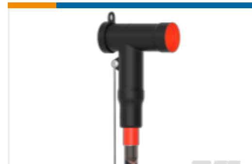
TE 产品编号CM0009-005 屏蔽式可分离连接器 1250 A
