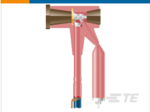
TE 产品编号414371-014 RICS 非绝缘 T 型适配器
